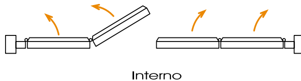
S13 1°, 2° e 4° Anta Semifissa - 2° Anta apribile a SX
